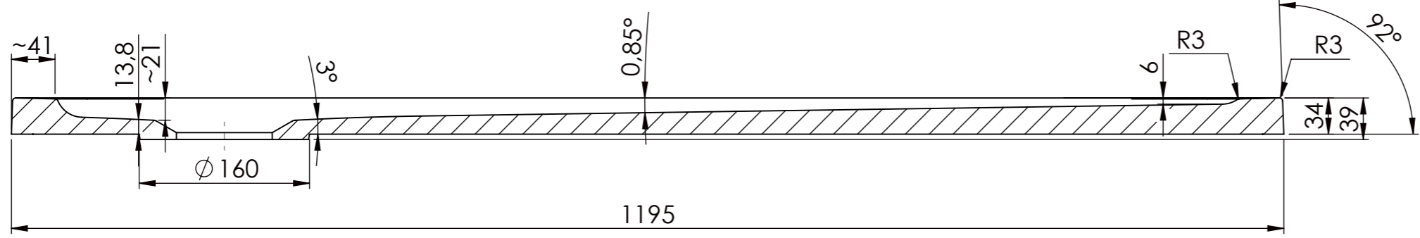
A-A (1:5)
